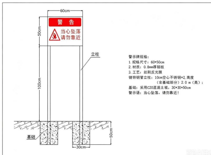
图 5-7 警示牌大样图②护栏工程
